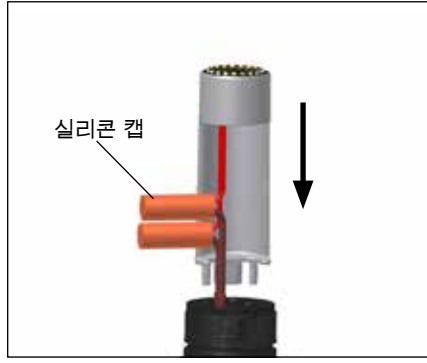
10. 실리콘 캡을 크립프 절연체 위로 밀어 넣습니다. 표시등 모듈을 익스페디터에 설치합니다.
