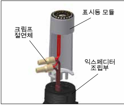
9. 크립프 절연체를 끼웁니다.
